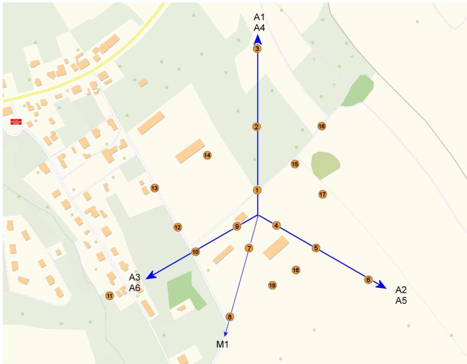
Zał. nr 1: Lokalizacja anten oraz ich azymuty, lokalizacja pionów (punktów) pomiarowych wokół instalacji radiokomunikacyjnej. ● -punkt (pion) ● pomiarowy.
