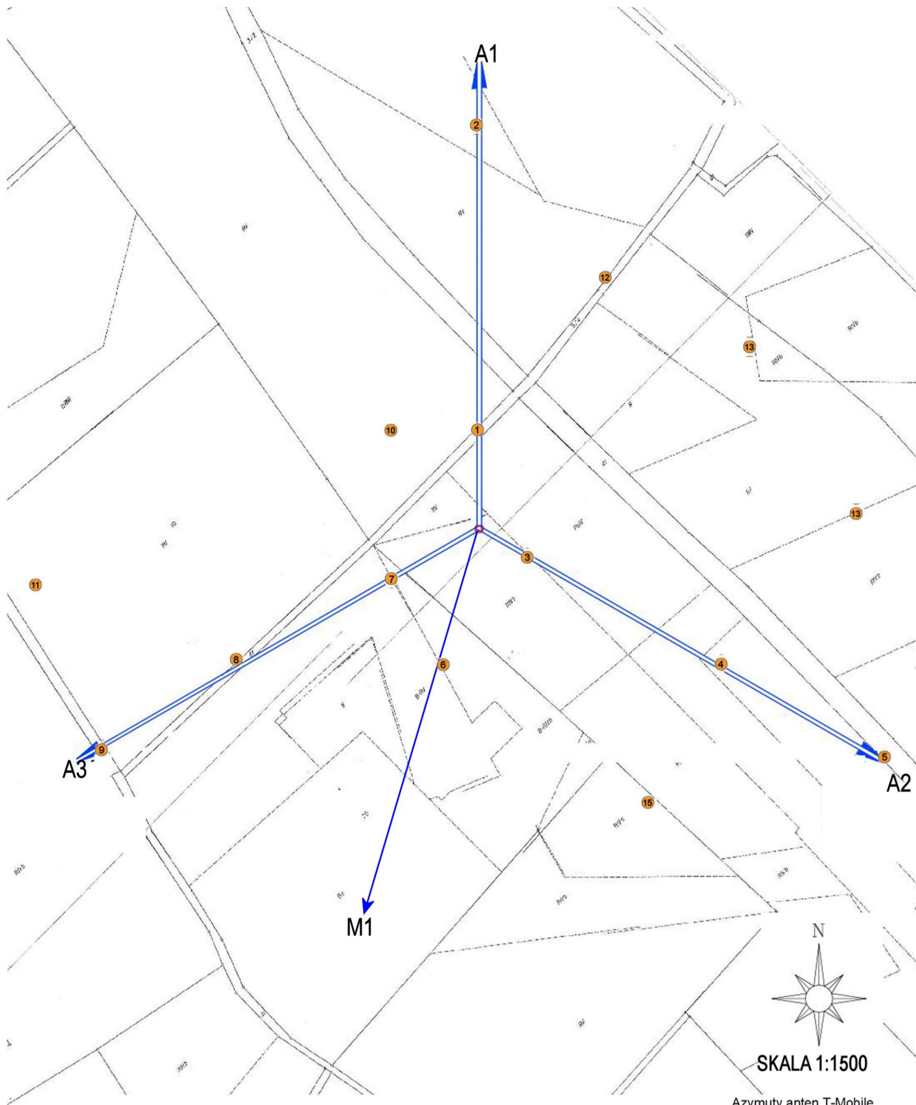
Azymuty anten T-Mobile
