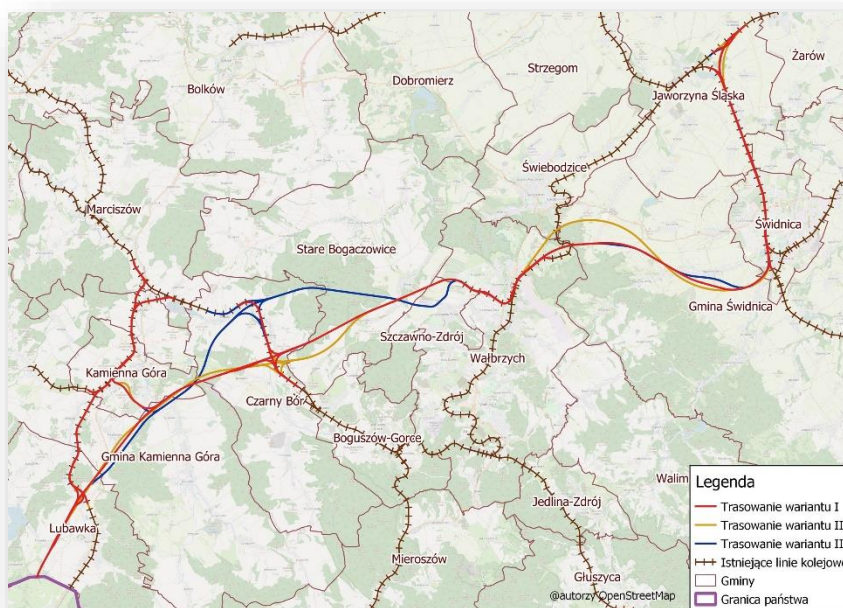
Rysunek 4. Możliwe warianty przebiegu linii kolejowej dużych prędkości.
