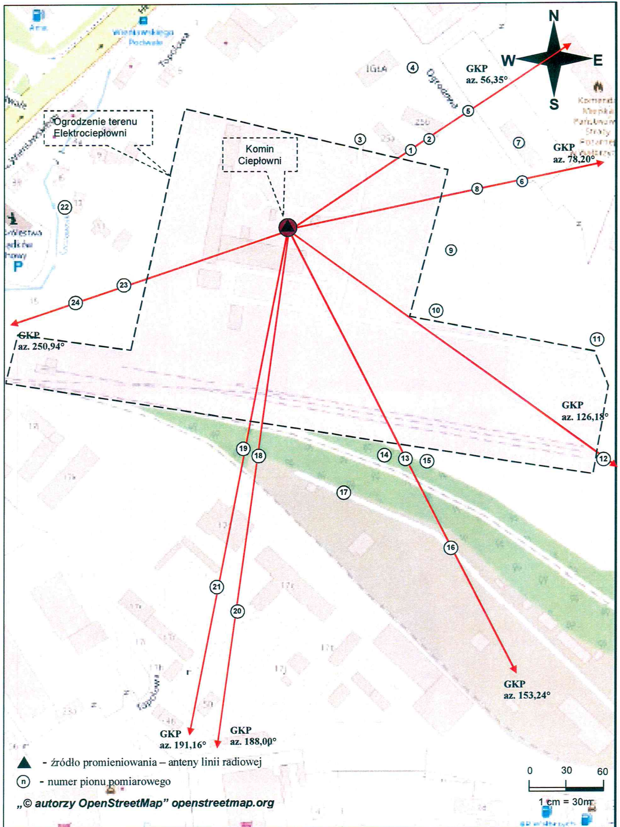
Rys. 1. Usytuowanie punktów i pionów pomiarowych w otoczeniu instalacji radiokomunikacyjnej Stacja Netia WALBD047-WALBM00011 Wałbrzych, ul. Ogrodowa 25
