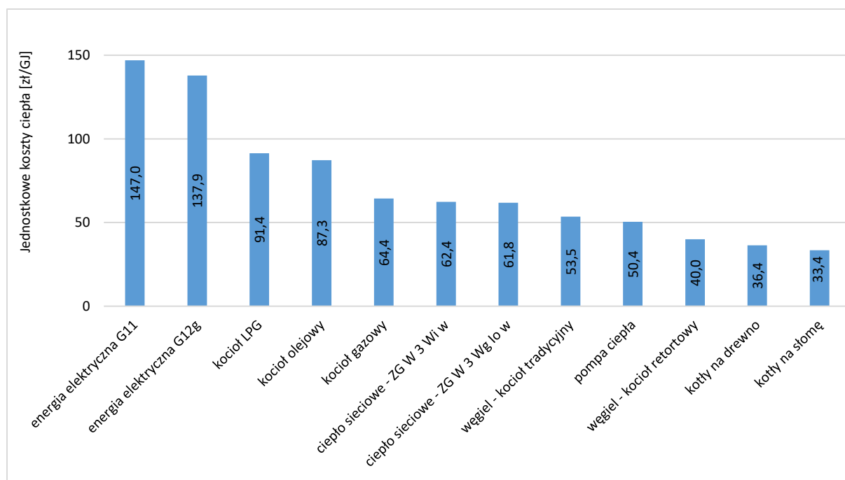
Rysunek 24 Porównanie rocznych kosztów wytworzenia energii w odniesieniu do jednostkowych wskaźników kosztów energii użytecznej dla różnych nośników
