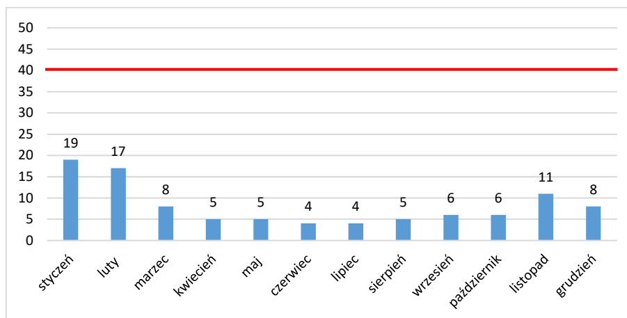
Rysunek 26 Stężenia średnioroczne dwutlenku azotu w 2017 r. na stacji w Wałbrzychu Źródło: opracowanie własne na podstawie danych ze strony air.wroclaw.pios.gov.pl/
