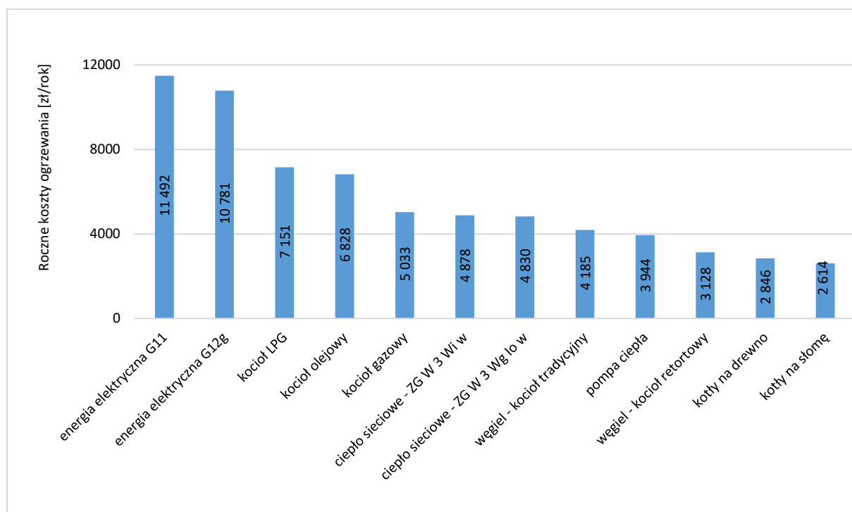
Rysunek 23 Porównanie kosztów wytworzenia energii w odniesieniu do energii użytecznej dla różnych nośników
