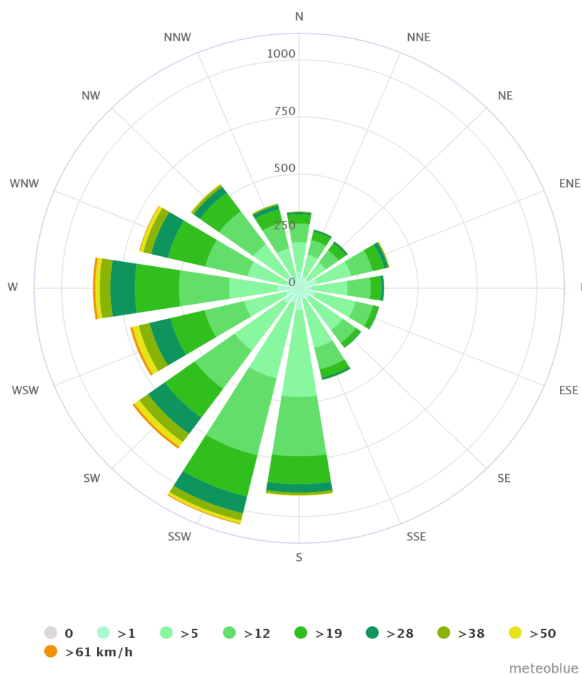
Rysunek 3 Róża wiatrów w rejonie Wałbrzycha Źródło: www.meteoblue.com
