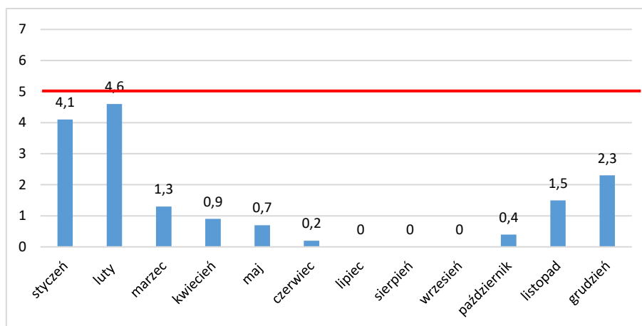
Rysunek 29 Stężenia średnioroczne benzenu w 2017 r. na stacji w Wałbrzychu Źródło: opracowanie własne na podstawie danych ze strony air.wroclaw.pios.gov.pl/
